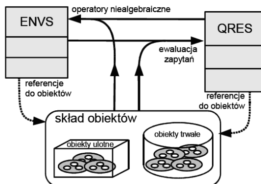
Rys. 1. Ewaluacja zapytań w obiektowych bazach danych opartych o podejście stosowe z wykorzystaniem stosów ENVS i QRES [1]
