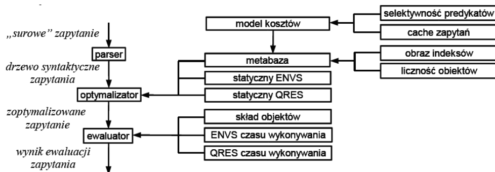
Rys. 3. Dynamiczny optymalizator zapytań dla SBQL jako rozbudowany optymalizator statyczny [9]
