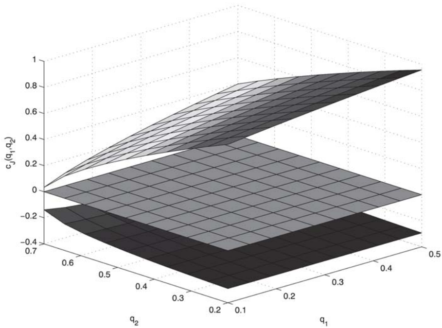
Rys. 3. Geometryczna interpretacja elementów macierzy wyjść C_j(q) w przestrzeni \mathbb{R}^3
