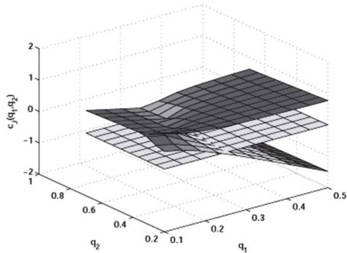
Rys. 6. Elementy macierzy wyjść C_f(q) w przestrzeni \mathbb{R}^3
