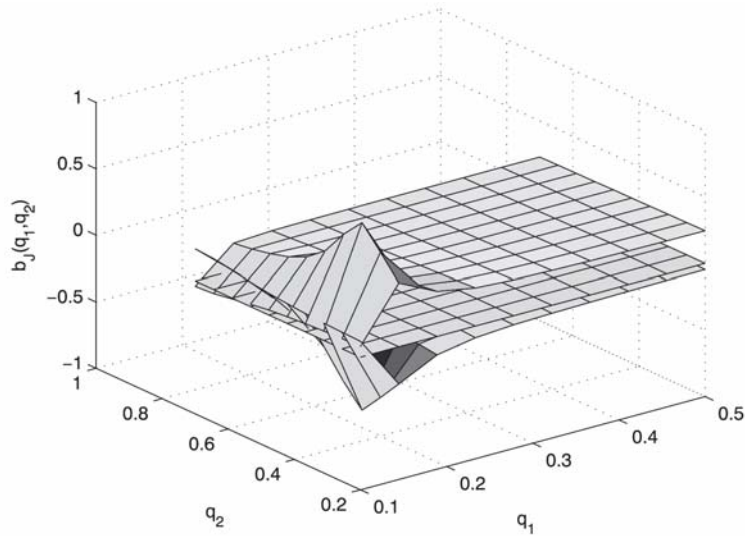
Rys. 5. Elementy macierzy sterowań B_f(q) w przestrzeni \mathbb{R}^3
