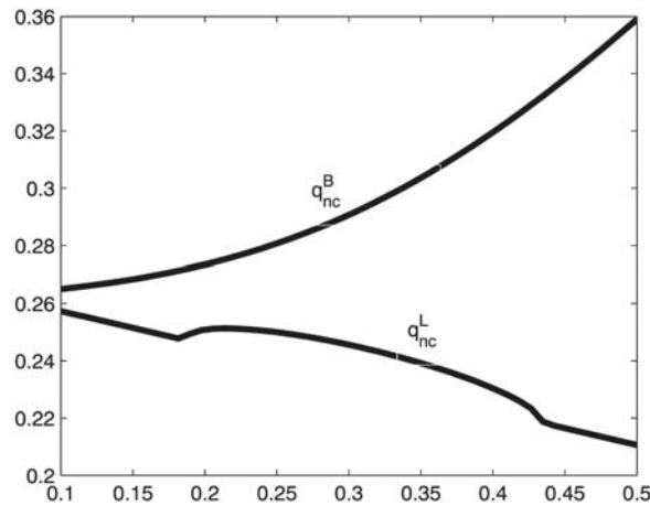
Rys. 8. Obszar niesterowalności Q_{nc} dla rozważanego przykładu
