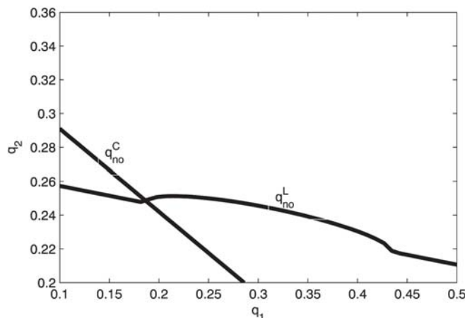
Rys. 9. Obszar nieobserwowalności Q_{no} dla rozważanego przypadku
