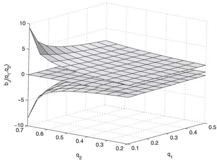
Rys. 2. Geometryczna interpretacja elementów macierzy sterowań B_j(q) w przestrzeni \mathbb{R}^3
