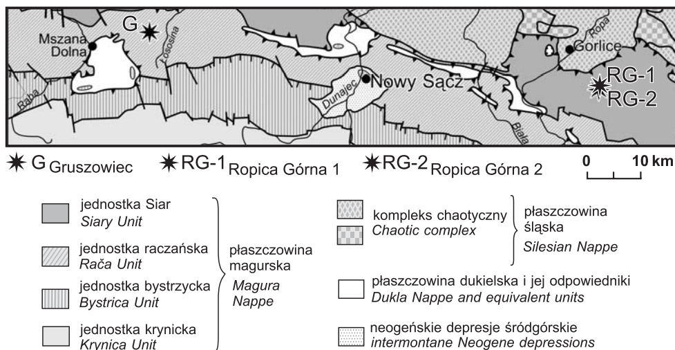
Fig. 1. Lokalizacja badanych odsłoneń w płaszczowinie magurskiej; geologia według Żytki et al. (1988) i Świerczewskiej (2005)
