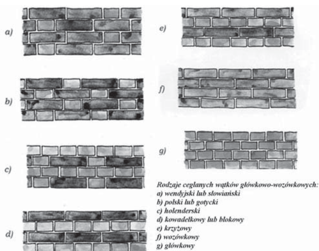
Rys. 11. Przykładowe wązki murów ceglanych
