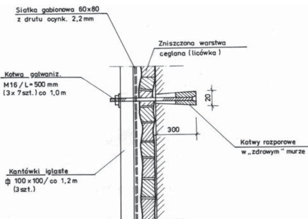
Rys. 9. Siatka gabionowa z drutu ocynkowanego
