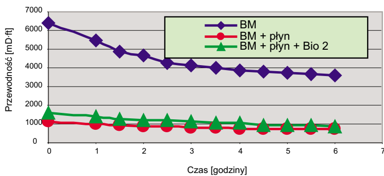
Rys. 4. Przewodność podsadzki BM 16/30 w temperaturze 50°C
