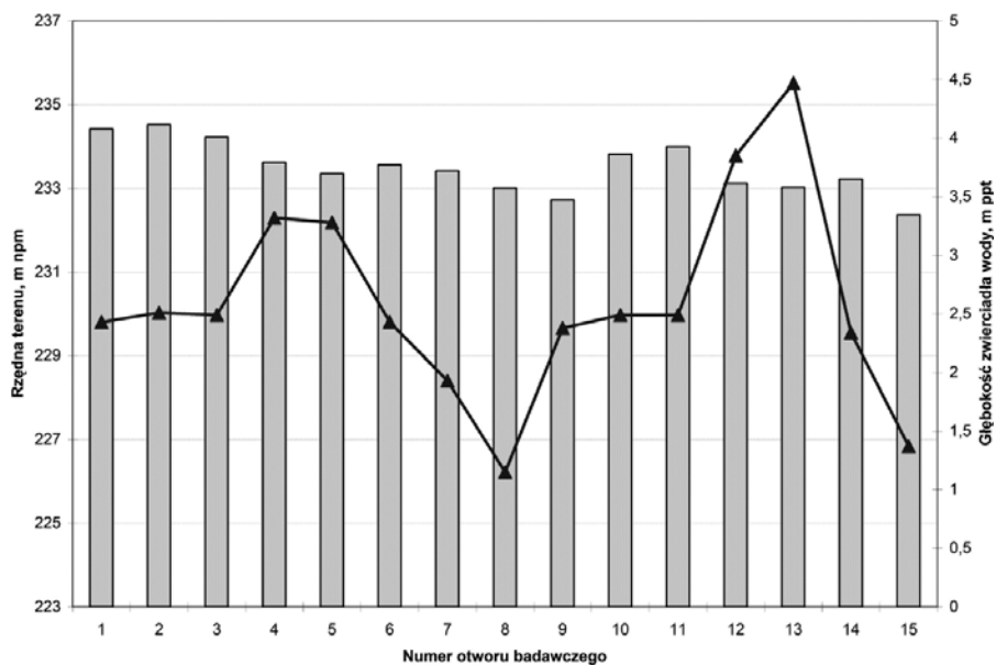
Rys. 2. Głębokość zwierciadła wody podziemnej i rzędna terenu
