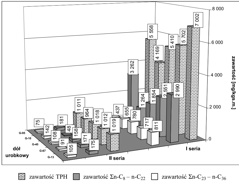
Rys. 2. Porównanie zawartości TPH, \Sigma n-C_8 - n-C_{22} , \Sigma n-C_{23} - n-C_{36} po zabiegach inokulacji biopreparatem (G-1) na bazie mikroorganizmów autochtonicznych (I seria) i biopreparatem (G-2) na bazie mikroorganizmów autochtonicznych i grzybów (II seria) na wytypowanych do badań dołach urobkowych
