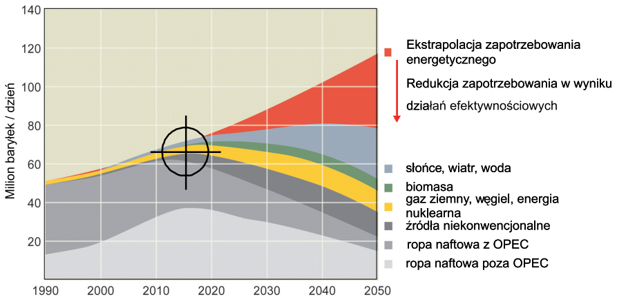
Rys. 1. Światowe zapotrzebowanie na energię wg prognoz International Energy Agency [1] Źródło: [Erdölprognose der IEA (International Energy Agency)]
