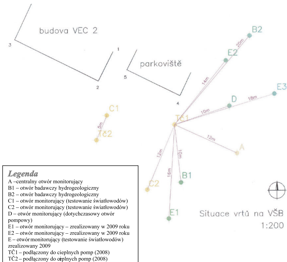
Rys. 1. Rozmieszczenie otworów badawczych w obrębie poligonu badawczego VSB-TU Osraua
