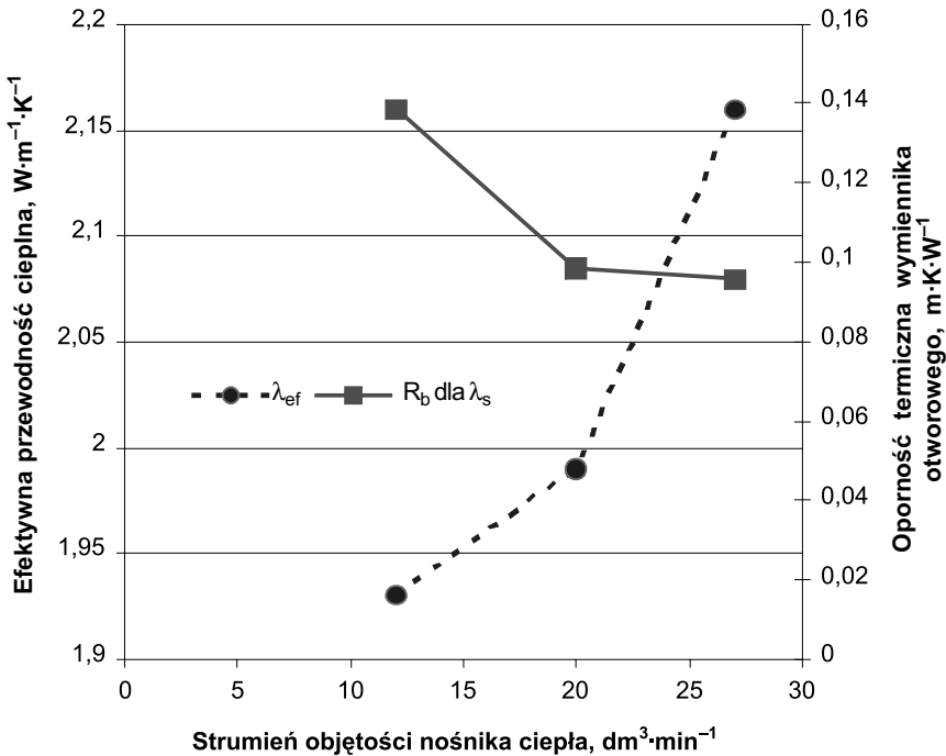
Rys. 10. Zależność efektywnej przewodności cieplnej w wymienniku otworowym nr 3 oraz oporności termicznej od strumienia objętości nośnika ciepła
