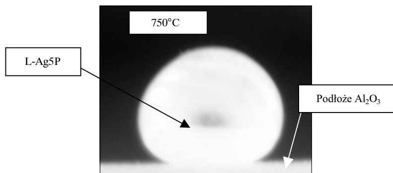
Rys. 3. Widok próbki L-Ag5P na niezwilżalnym podłożu \text{Al}_2\text{O}_3
