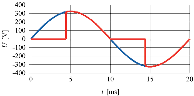
Rys. 1. Sterowanie triakiem
