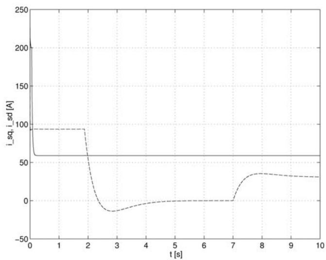
Rys. 11. Przebieg prądów i_{sq} (---) i i_{sd} (—) przy rozruchu i stabilizacji silnika – bez filtracji wartości zadanej
