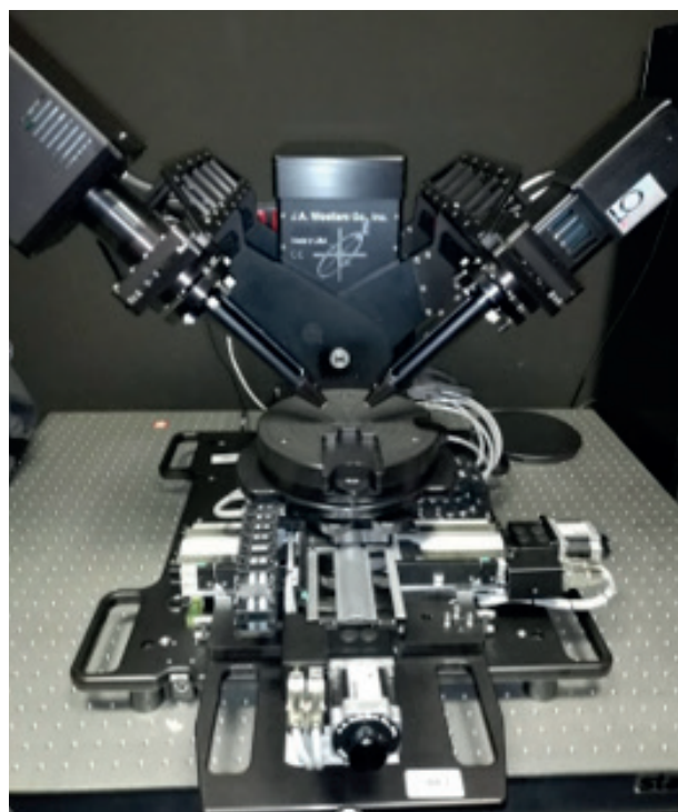
Rys. 7. Elipsometr spektroskopowy Wollam 2000
