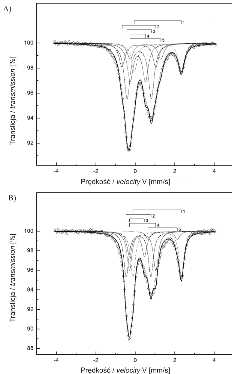
Fig. 4. Widma mössbauerowskie: A) sepiolitu żelazowo-żelazowego; B) saponitu żelazowo-żelazowego z diabazów z Niedźwiedziej Góry. 1–5 – numery linii składowych widm; odpowiadające im parametry zestawiono w tabeli 3
