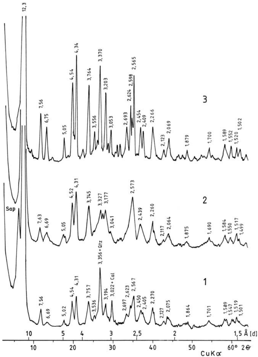
Fig. 3. Dyfraktogramy rentgenowskie sepiolitów: 1 – żelazowo-żelazawego z diabazów z Niedźwiedziej Góry, 2 – magnezowego z tzw. melafirów z Rudna, 3 – magnezowego z marmurów dolomitowych z Rędzin. Symbole refleksów pochodzących od domieszek: Cal – kalcyt, Qtz – kwarc, Sap – saponit, + – koincydencja z refleksami sepiolitu
