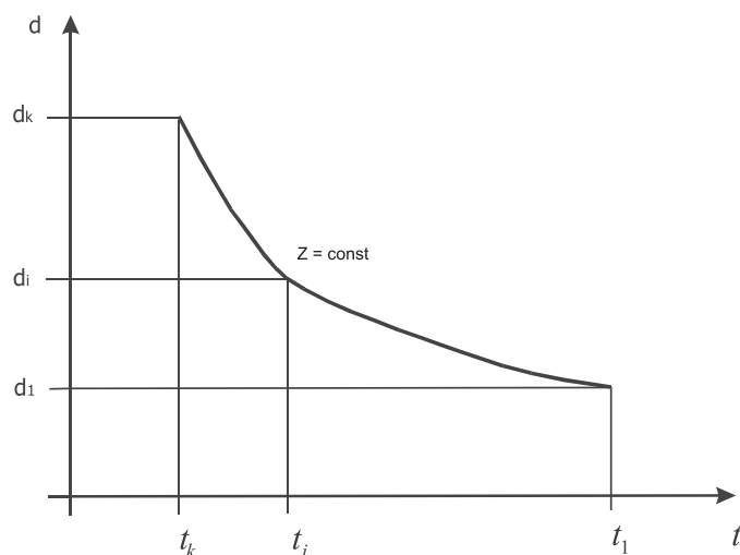
Rys. 5. Zależność kroku całkowania od średnicy kropli
