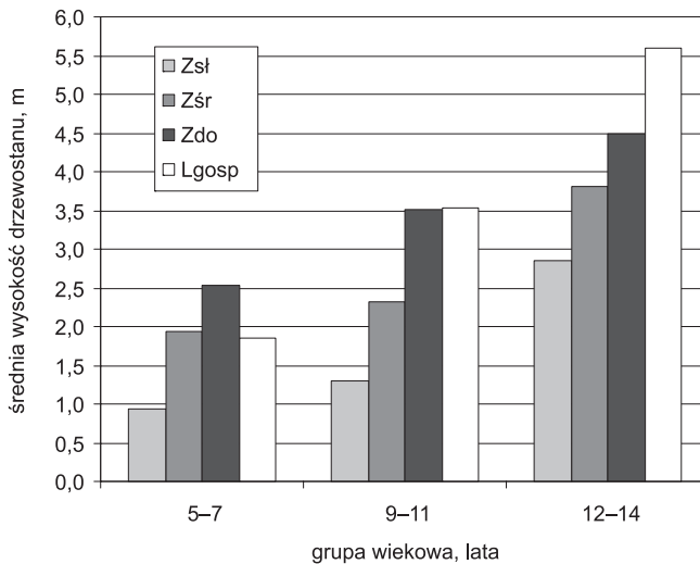
Rys. 1. Wysokość sosny na zwałowisku zewnętrznym KWB „Bełchatów” w porównaniu do sosny w gospodarczych drzewostanach na siedlisku boru mieszanego świeżego (BMśw) w zależności od wieku z podziałem na grupy wzrostowe, gdzie: Zsł — powierzchnie na zwałowisku o wzroście słabym; Zśr — średnim; Zdo — dobrym; Lgosp — powierzchnie porównawcze w drzewostanach gospodarczych
