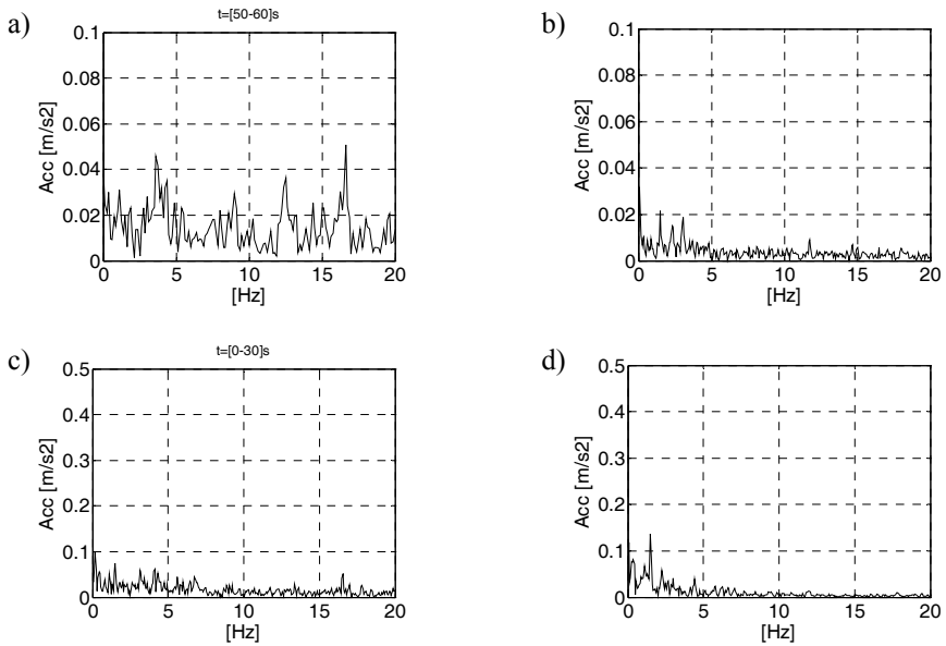
Rys. 9. Widma obwiedni dla przekładni w prawidłowym (good — G) i nieprawidłowym (bad — B) stanie technicznym dla: a)–b) niewielkiego obciążenia (G, B); c)–d) duże obciążenia (G, B)
