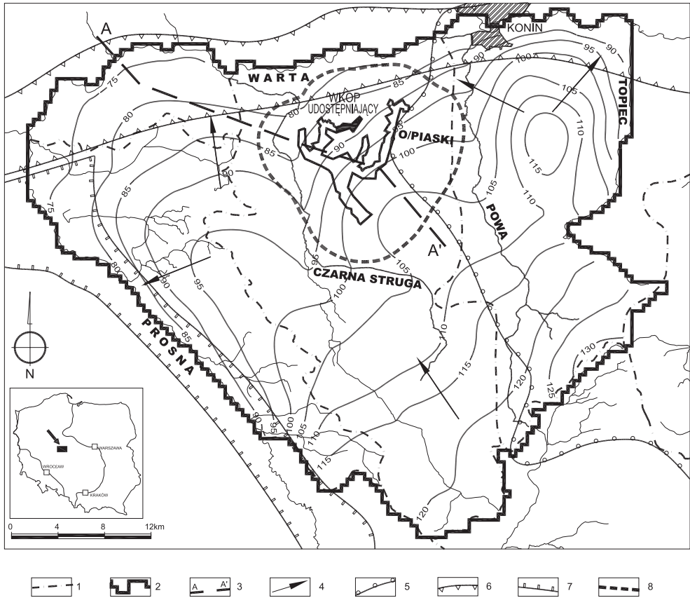
Rys. 1. Mapa hydroizohips [m n.p.m.] poziomu II w rejonie złoża „Piaski” w warunkach naturalnych: 1 — granice wododziałów, 2 — granica modelu matematycznego, 3 — przekrój hydrogeologiczny A-A', 4 — główne kierunki przepływu wód podziemnych, 5 — zasięg GZWP nr 151, Turek – Konin – Koło [4], 6 — zasięg GZWP nr 150, Pradolina Warszawsko-Berlińska, 7 — Zasięg GZWP nr 311, Zbiornik rzeki Proсна, 8 — prognozowany maksymalny zasięg izoliny depresji s = 1 m,
