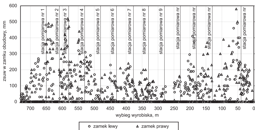
Rys. 2. Wykres wielkości zsuwów w zamkach odrzwi obudowy stalowej łukowej podatnej
