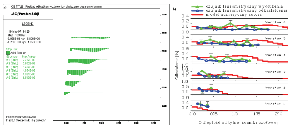
Rys. 4. Rozkład odkształceń w zbrojeniu po wykonaniu konstrukcji — obciążenie ciężarem własnym(a); porównanie wyników odkształceń zbrojenia po wykonaniu konstrukcji (b)
