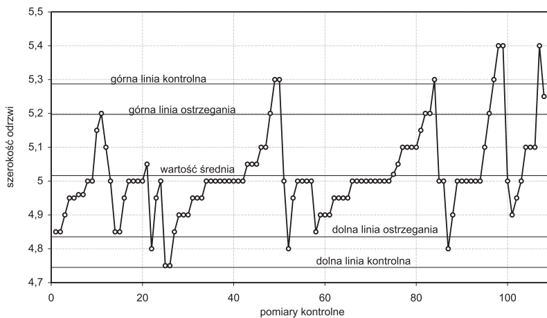
Rys. 1. Przykład karty kontrolnej szerokości stalowej obudowy odzwiowej [1]
