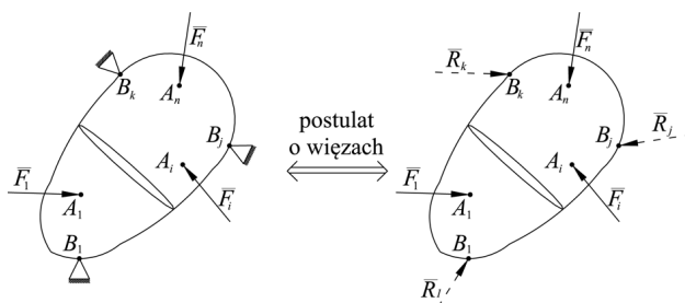
Rys. 5. Układ sił działający na ciało sztywne
