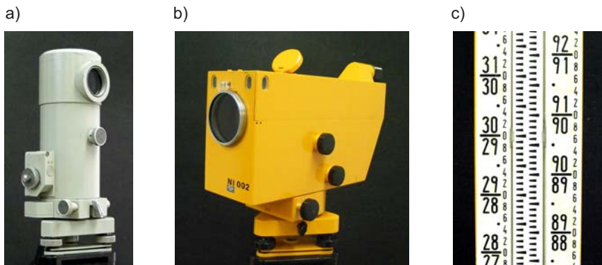
Rys. 1. Niwelatory precyzyjne optyczne: a) Ni 007, b) Ni 002 oraz c) fragment łaty inwarowej
