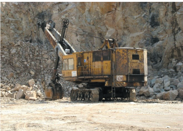
Rys. 9. Jednonaczyniowa linowo-elektryczna koparka przedsiębiorna Skoda E-303
