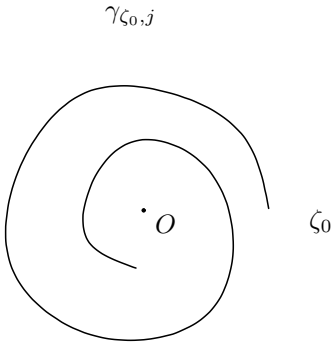
Fig. 3. \beta_j > 0
