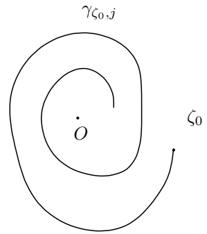
Fig. 4. \beta_j < 0
