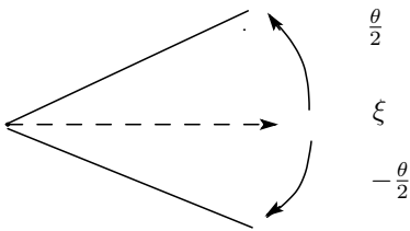
Fig. 1. S_{\theta,\xi}
